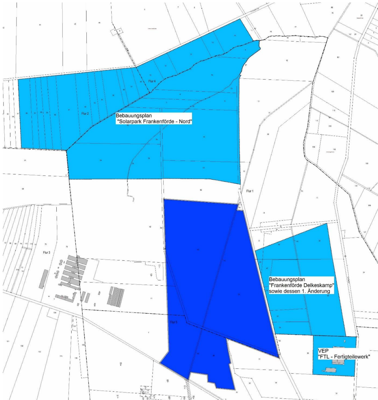
Abb.6: Benachbarte Bebauungspläne (@GeoBasis-DE/LGB 2022)
