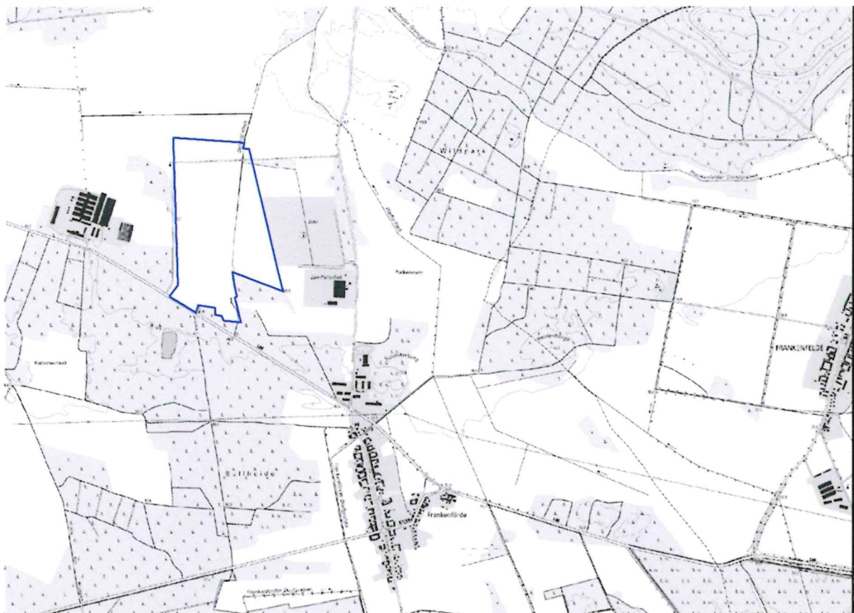
Lage des Plangebietes (8. Änderung des Flächennutzungsplanes der Gemeinde Nuthe-Urstromtal im Bereich des Bebauungsplanes Frankenförde Nr. 6 „Solarpark Frankenförde-An der L 80“)
