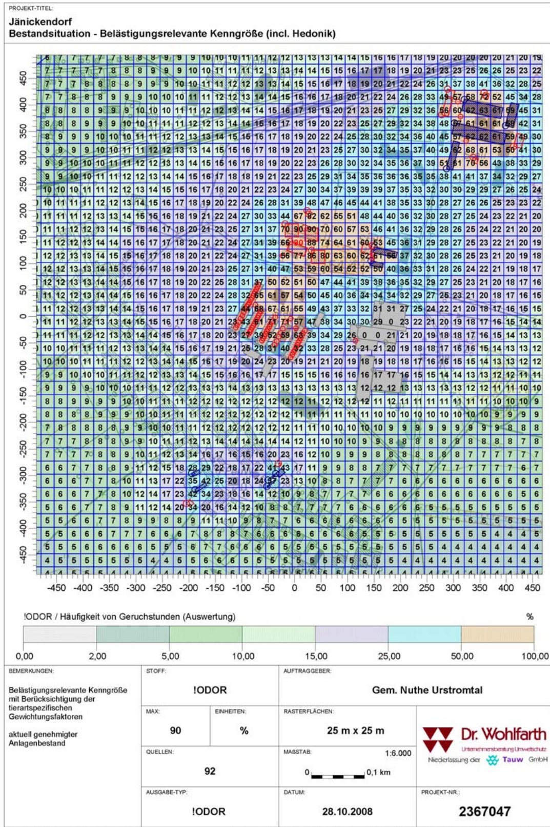
Abbildung 4.3: Belastungsrelevante Kenngröße berechnet mit aktuellen Bestandsdaten und aktualisierten Emissionsfaktoren
